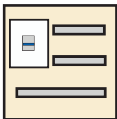
DIN/3 & DINS/3 2x12+1x24 = 48 mód.+ICP
