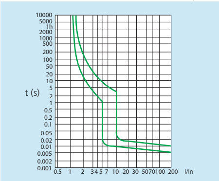
Curva C para CA
