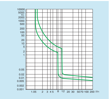
Curvas según UNE-EN 60947-2
