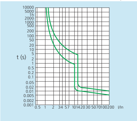
Curva 7-15 para CC
