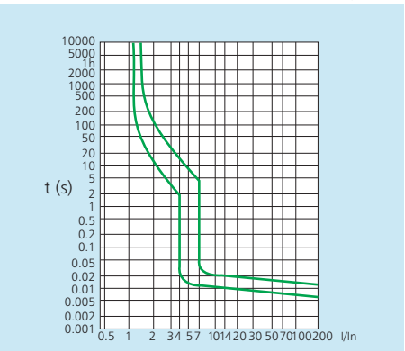
Curva 4-7 para CC
