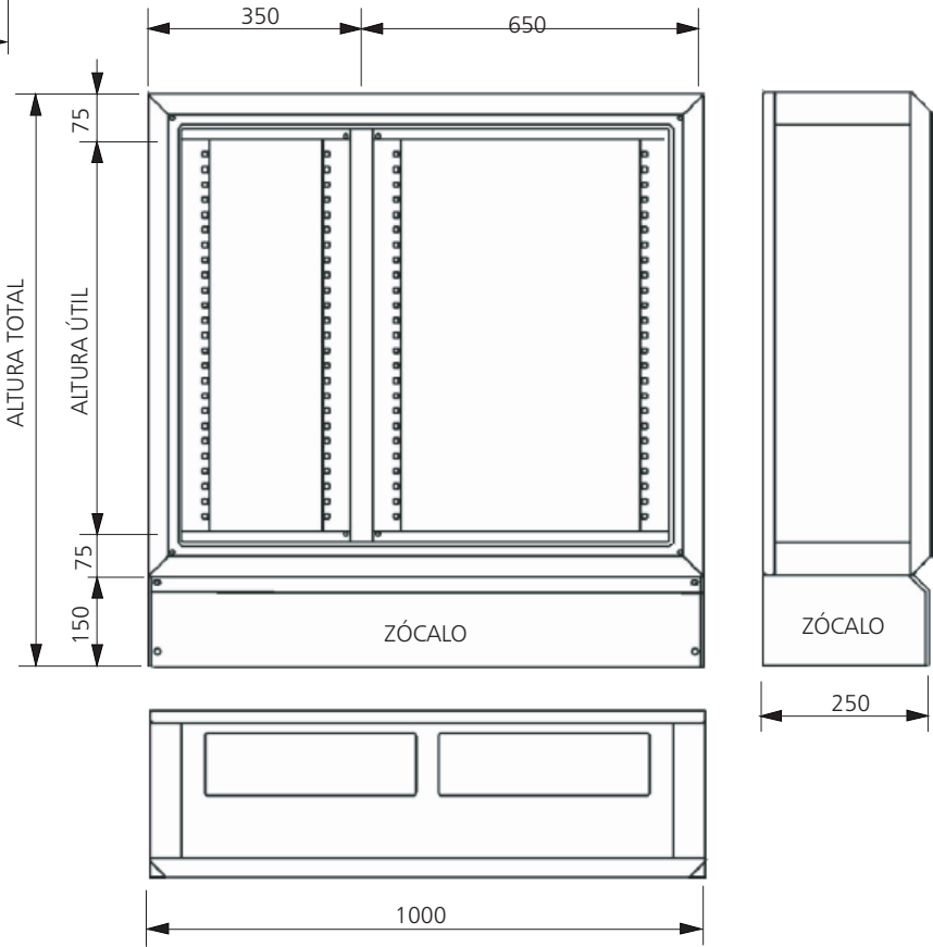
ARMARIOS DE ALTURA: 1650, 1950mm (más zócalo)
